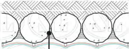
預壘樁工法
